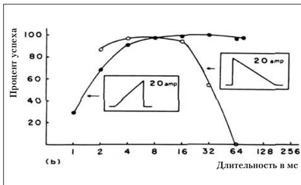
Рис. 4. Зависимость процента успеха вентрикулярной дефибрилляции от длительности треугольных импульсов с инкрементом и декрементом затухания и амплитудой тока 20 А. Schuder et al. [17,18].
